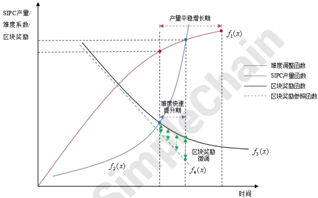
图 12 SIMPLE 函数图
